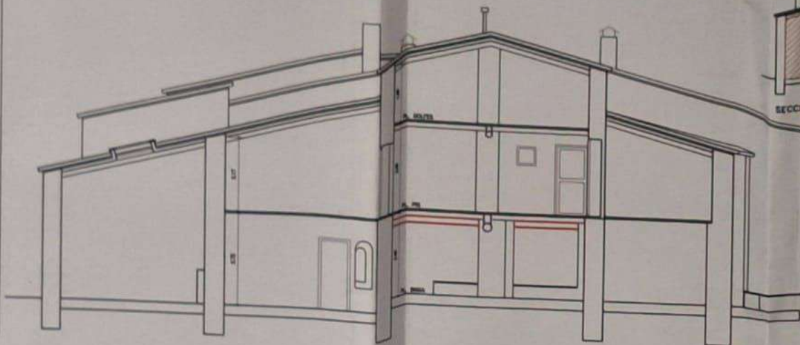
SECCIÓ A-A'
