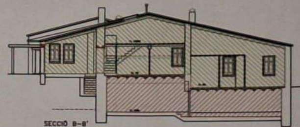
SECCIÓ B-B'
