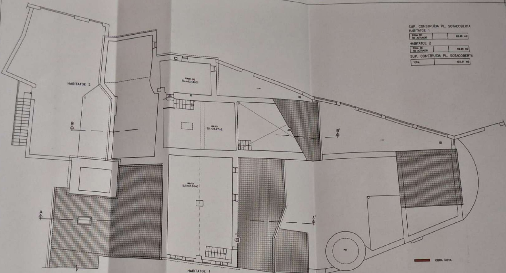
PLANTA SOTACOBERTA ESCALA 1/100
