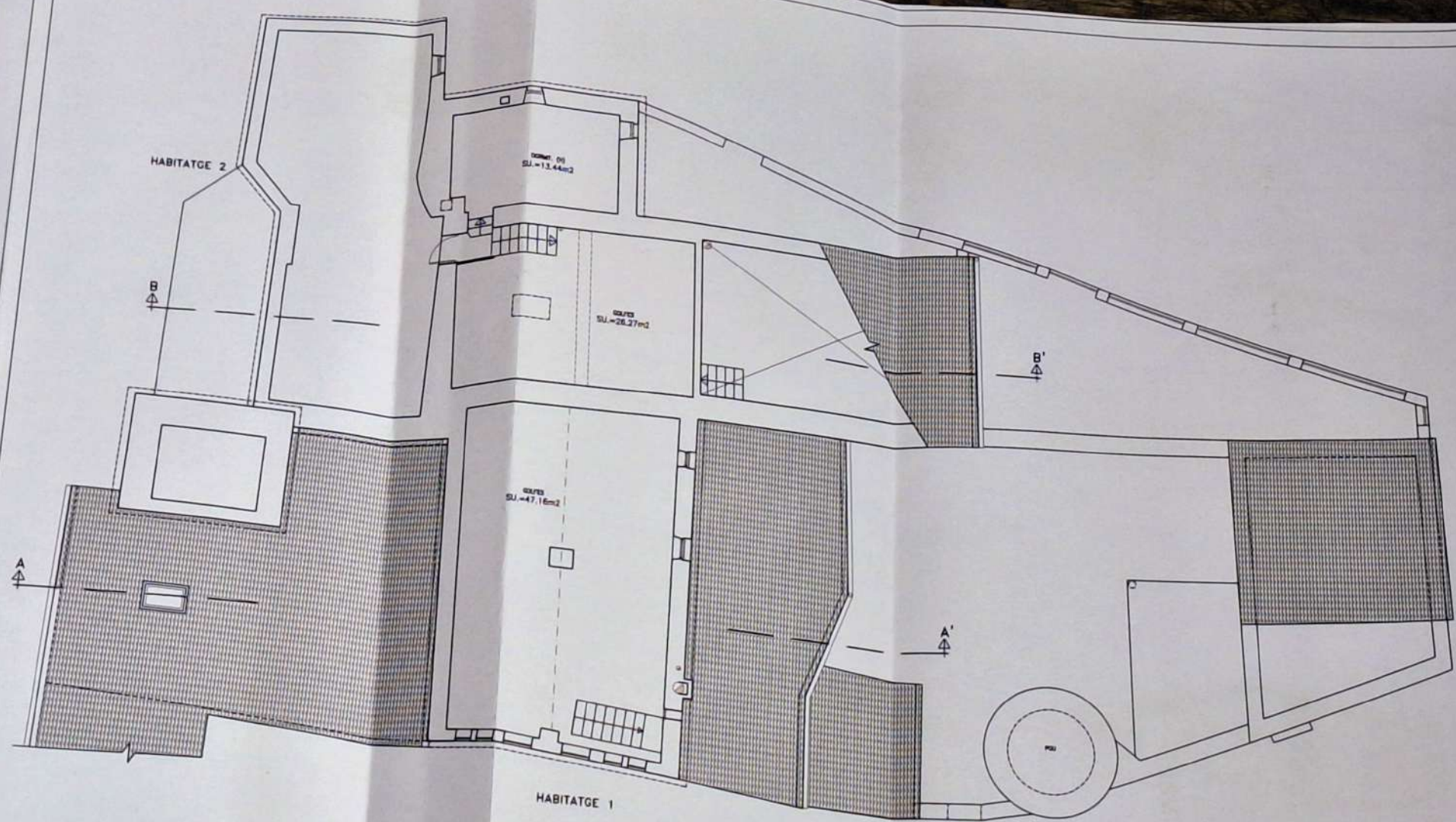
PLANTA SOTACOBERTA
